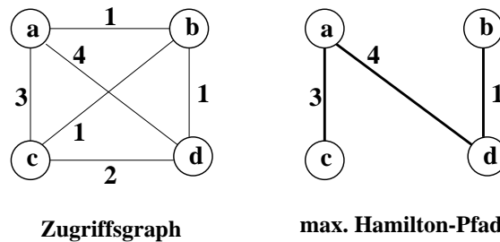
Abbildung 5: Graphmodell zur Adreßoptimierung für skalare Variablen
