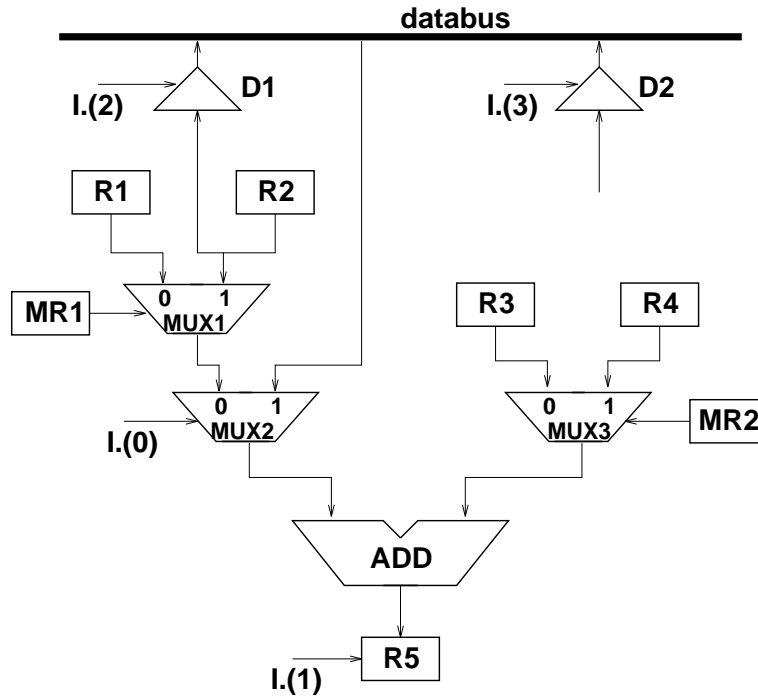
Abbildung 3: Partielle Prozessorstruktur auf Register-Transfer-Ebene
