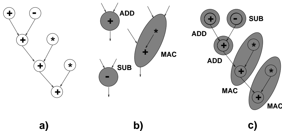
Abbildung 4: Befehlsauswahl: a) Ausdrucksbaum, b) Baumdarstellung der Maschinenbefehle, c) optimale Überdeckung
