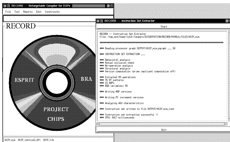
Abbildung 2: Das RECORD-System: Benutzeroberfläche und Befehlssatz-Extraktor
