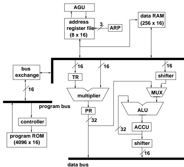
Abbildung 1: Vereinfachte Architektur eines Texas Instruments TMS320C25 DSP. Die Spezialregister TR, PR und ACCU können teilweise parallel beschrieben werden. Ebenso kann die spezielle Adreßrecheneinheit (AGU) parallel zum übrigen Rechenwerk betrieben werden.
