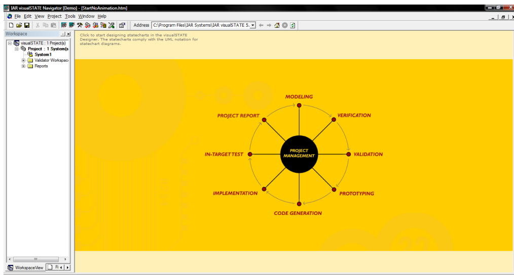
Abbildung 1: Hauptbildschirm
